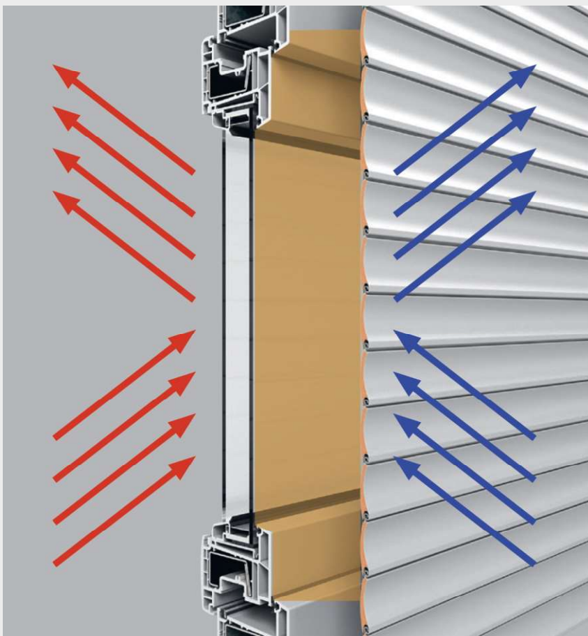
Die Luftschicht zwischen Fenster und Rollläden wirkt wärmedämmend und hilft, Heizkosten zu senken.
